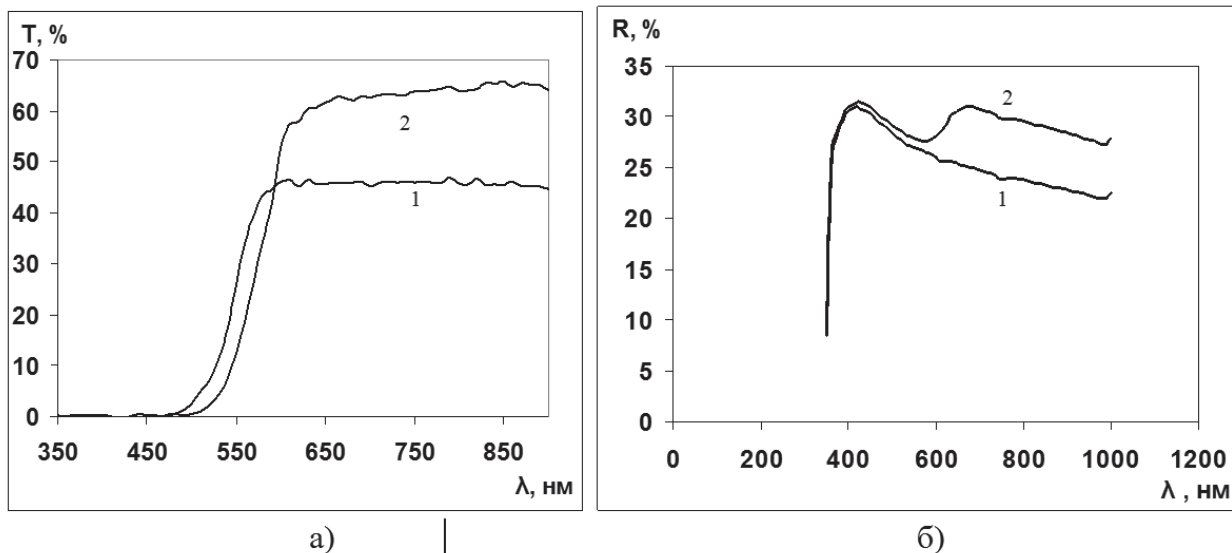
Рис. 1. а) Спектральная зависимость коэффициента пропускания пленок V_2O_5 . б) Спектры отражения пленок V_2O_5 . 1 – исходная пленка, 2 – модифицированная в результате электрополевого воздействия. Толщина пленки 2,95 мкм
