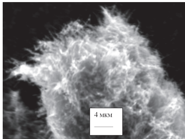
Рис. 3. Микрофотография одного из образцов волокна после очистки
