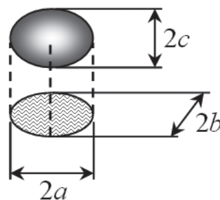
Рис. 4. Проекция модельной частицы на горизонтальную плоскость
