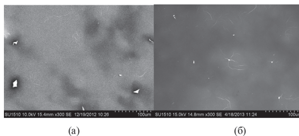
Рис. 4. Электронно-микроскопическое изображение пленки пентаоксида ванадия, полученное распылением из пульверизатора. Увеличено в 300 раз: а) исходный образец, б) окрашенная пленка
