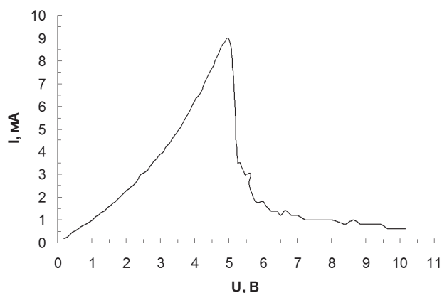
Рис. 2. Характерная вольт-амперная характеристика одного из исследуемых образцов
