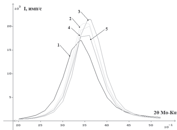
Рис. 2. Интенсивности рассеяния первого максимума на кривой распределения интенсивности для пленки пентаоксида ванадия: 1 – исходной, 2 – непосредственно после окрашивания, 3–5 – через 2, 4, 10 суток соответственно
