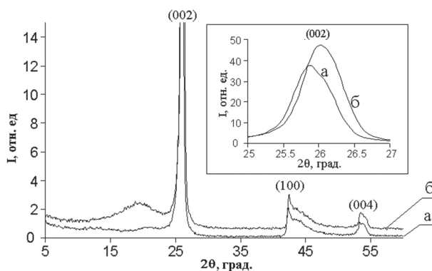
Рис. 4. Рентгеновские дифрактограммы волокон депозита: а) в исходном состоянии, б) после термообработки токопрохождением. На врезке представлен рефлекс (002) в увеличенном масштабе
