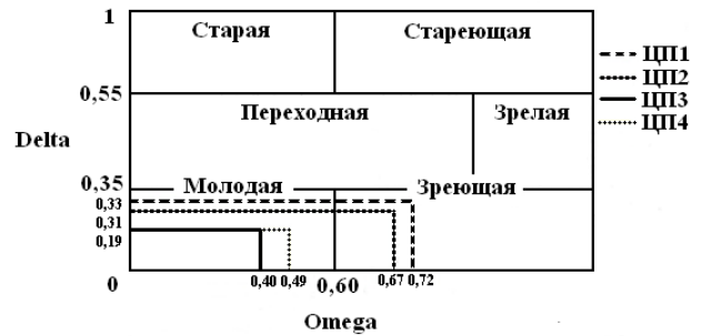
Рис. 3. Типы нормальных популяций, выделяемые критерием «дельта-омега»
